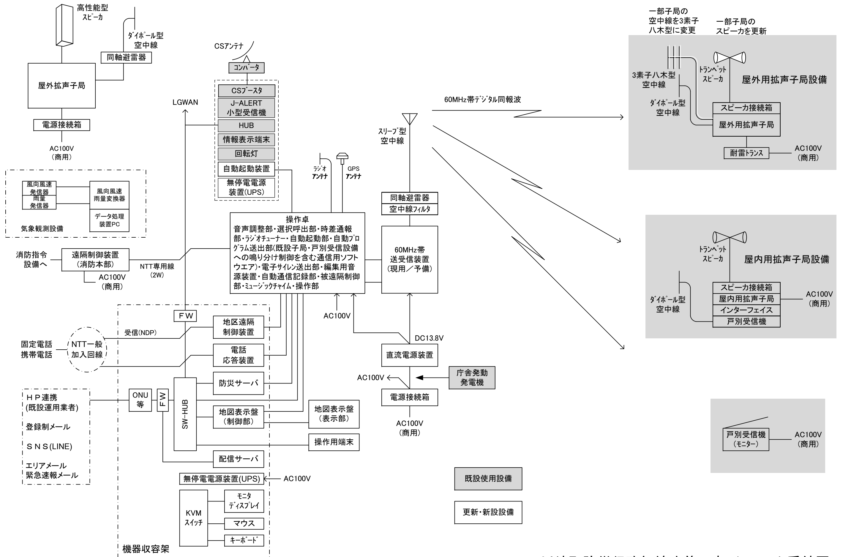
川崎町防災行政無線改善工事 システム系統図
